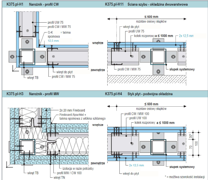
Detale, skala 1:5 Przekroje poziome - przykłady
